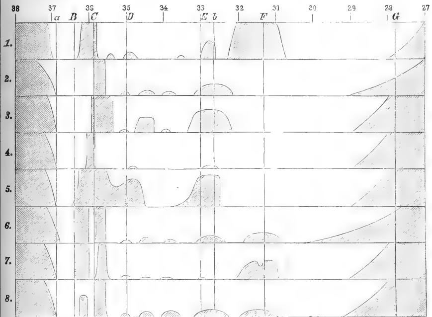
Fig. 3. Spectren des Bonelleins und seiner Derivate.
